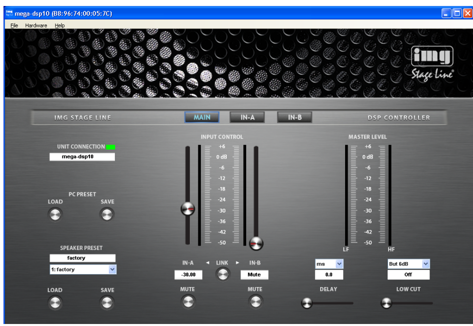
5) Hauptfenster für die Konfiguration eines Lautsprechers
